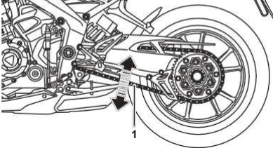
1. Maksimum dikey hareket konumu
